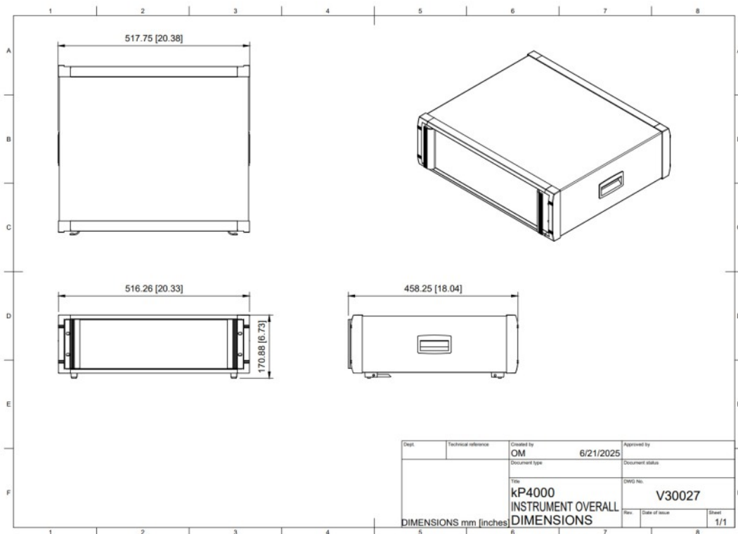
KP4110 Dimensions
