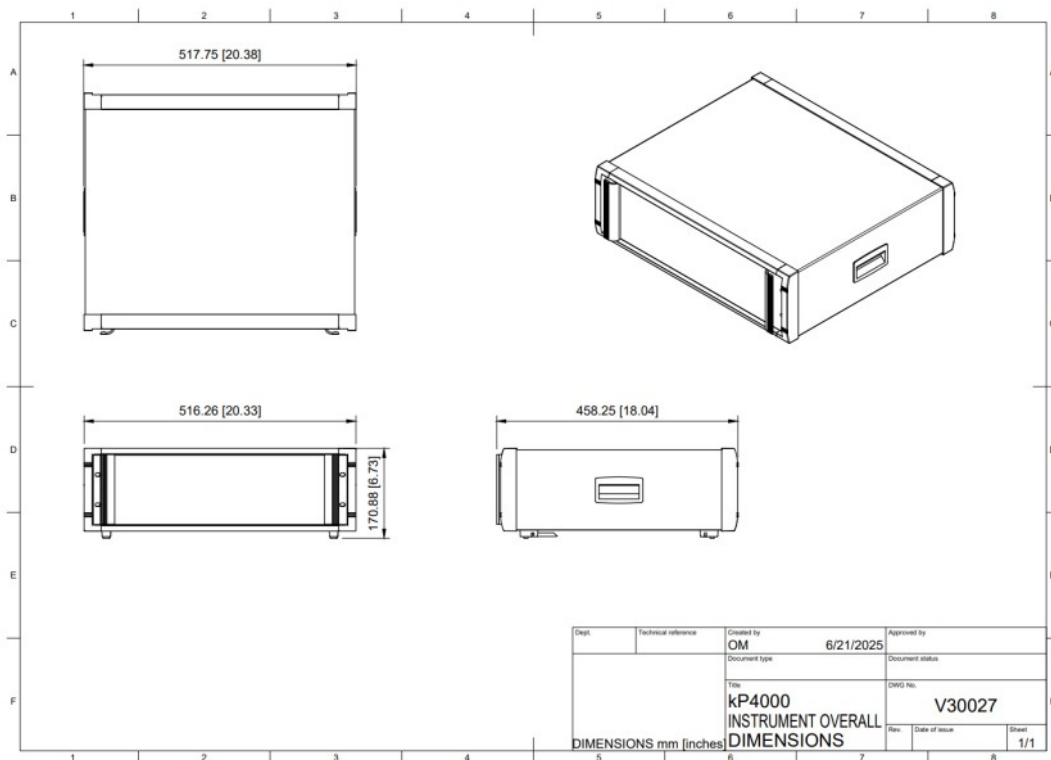
KP4106 Dimensions
