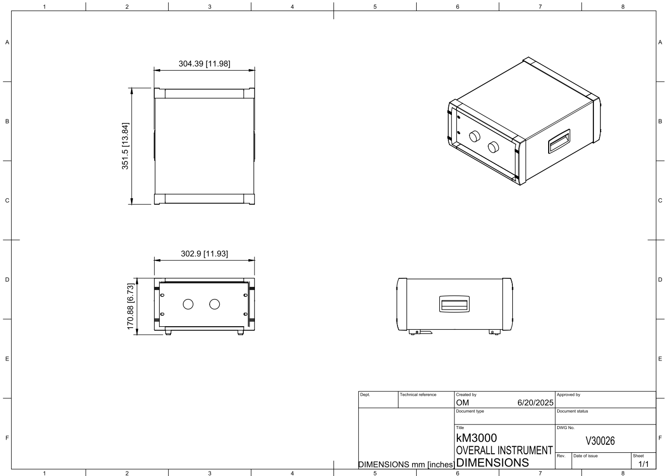
kM 3110 Dimensions
