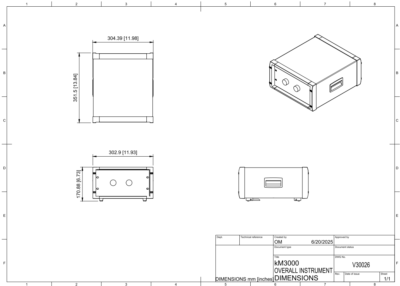
kM 3101 Dimensions
